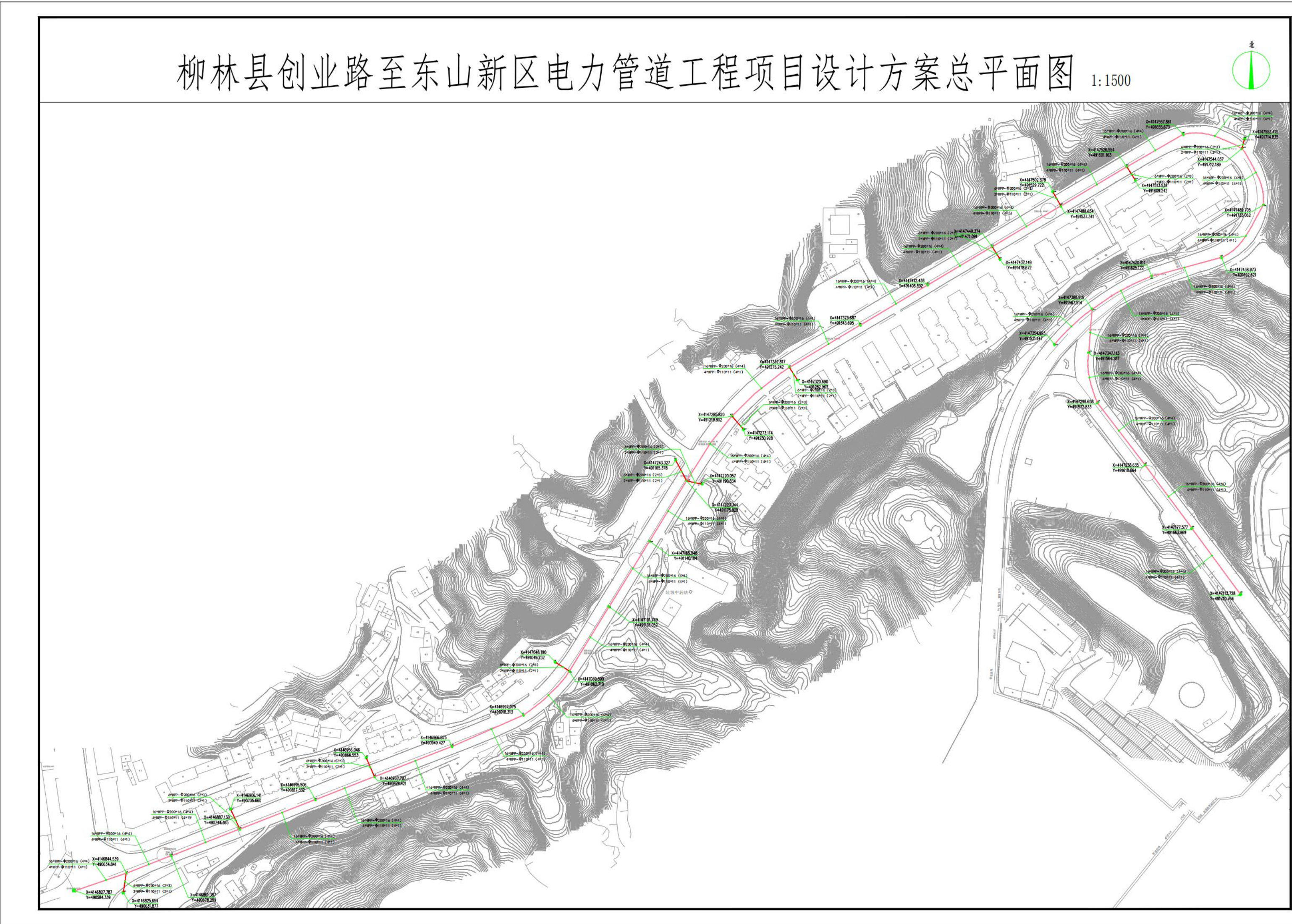
柳林县创业路至东山新区电力管道工程项目方案总平面图
