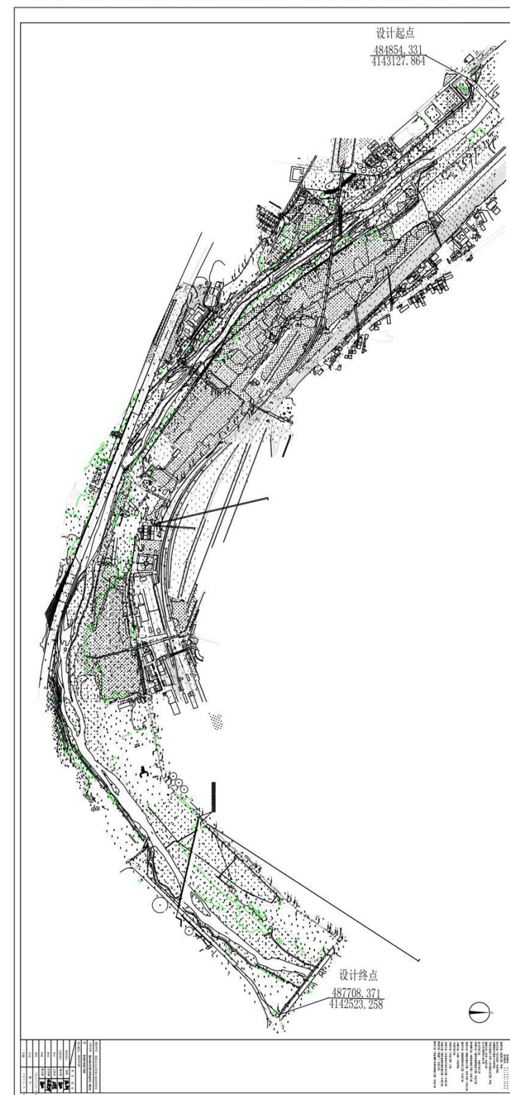
柳林县城区老旧燃气管网改造项目（穆村段）建设项目总平面图
